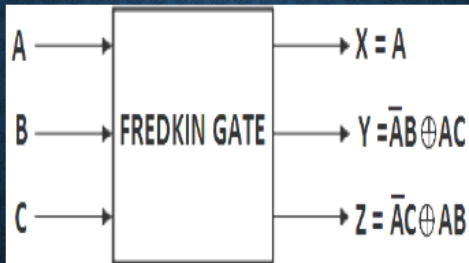
Fig. 7 Fredkin gate
